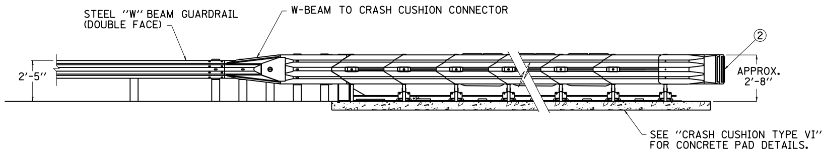
~ ELEVATION ~
