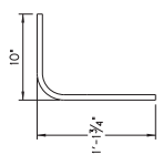
TYPE 3 BAR
