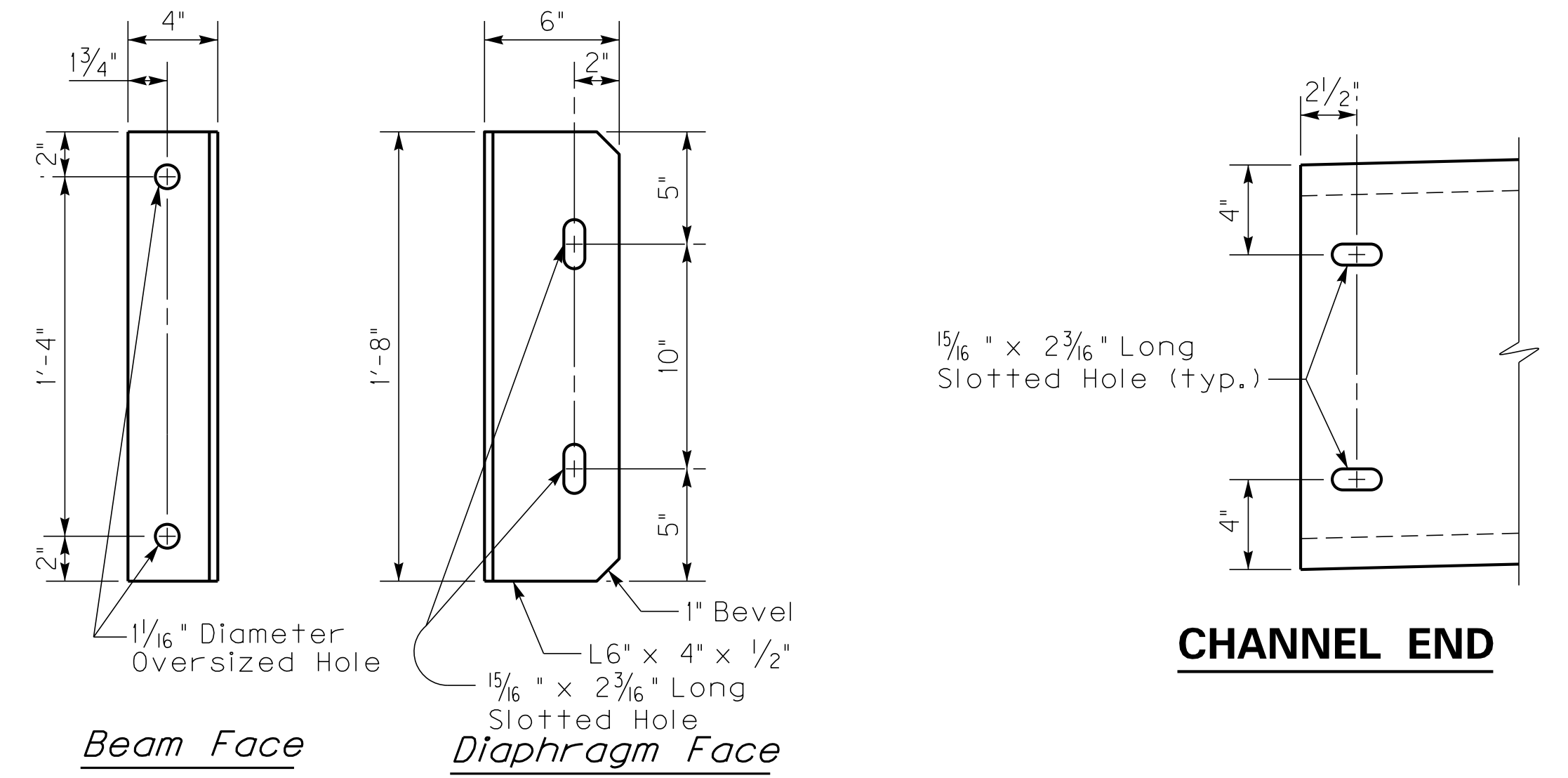
CLIP ANGLE - L1
