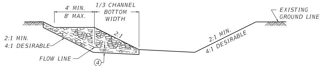
SECTION D-D
