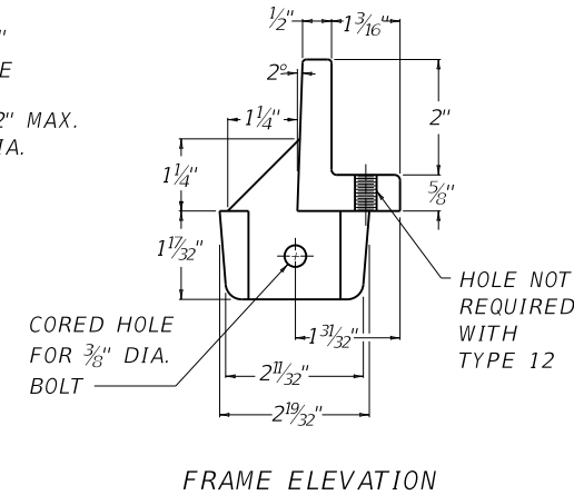
FRAME ELEVATION
