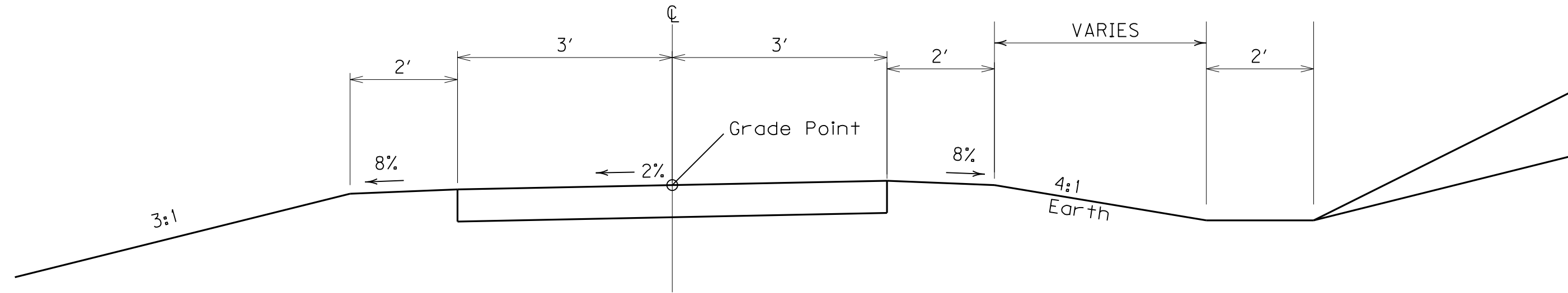
PEDESTRIAN PATH STA 4+08.09 TO STA 6+11.94
