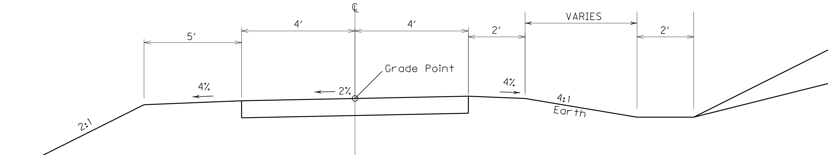
PEDESTRIAN PATH STA 0+19.73 STA 2+41.09
