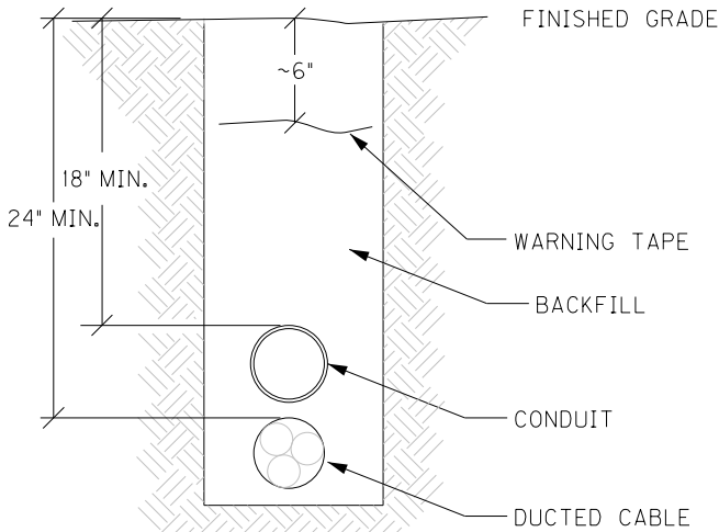
CONDUIT TRENCH
