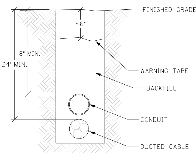
CONDUIT TRENCH
