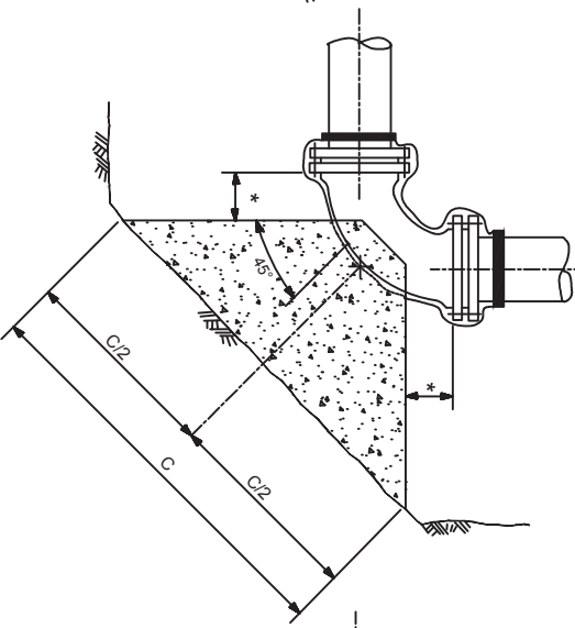
90° BEND
