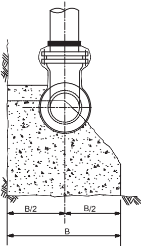
ELEVATION
