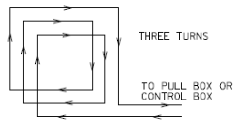
WIRING PLAN
