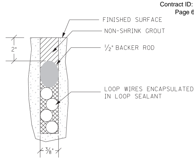
SECTION A-A (CONCRETE)
