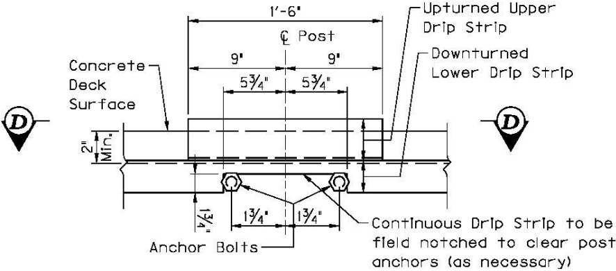
VIEW A-A
