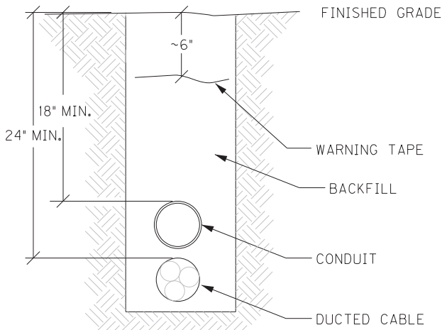
CONDUIT TRENCH
